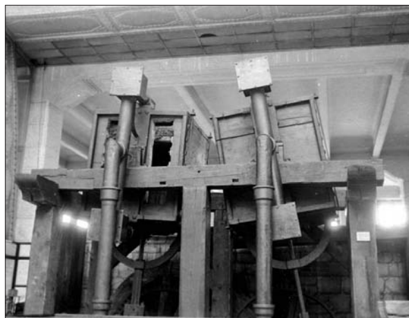
Vetrila savskega plavža (fotoarhiv GMJ).
