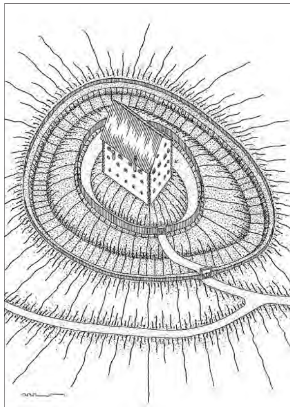
Variantna poskusa hipotetične rekonstrukcije nekdanje podobe gradu Žamberk. Aksonometrični študiji (risal: Igor Sapač, 2016 in 2021).
