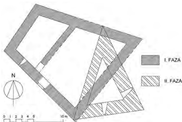
Shema tlorisne zasnove jedra kompleksa gradu Šalek s prikazom prve in druge faze stavbnega razvoja gradu v prvi in drugi polovici 13. stoletja (risal: Igor Sapač, 2016).
