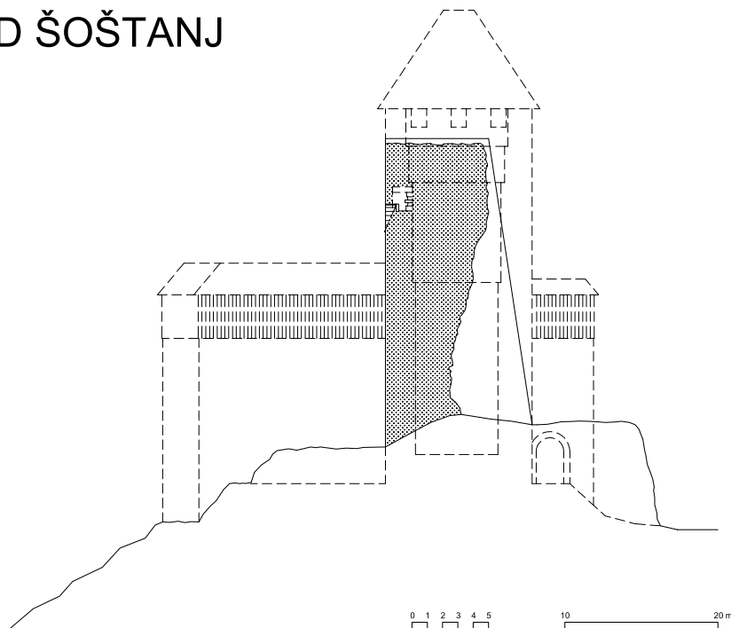
Poskus rekonstrukcije osnovne zasnove zahodne fasade gradu Šoštanj okoli leta 1200 s črtkano označenimi porušenimi deli in pikčasto označenim obsegom ohranjenega dela zahodne stene glavnega stolpa. Posebej je v prerezu narisano stranišče v severni steni stolpa (risal: Igor Sapač, 2021).
