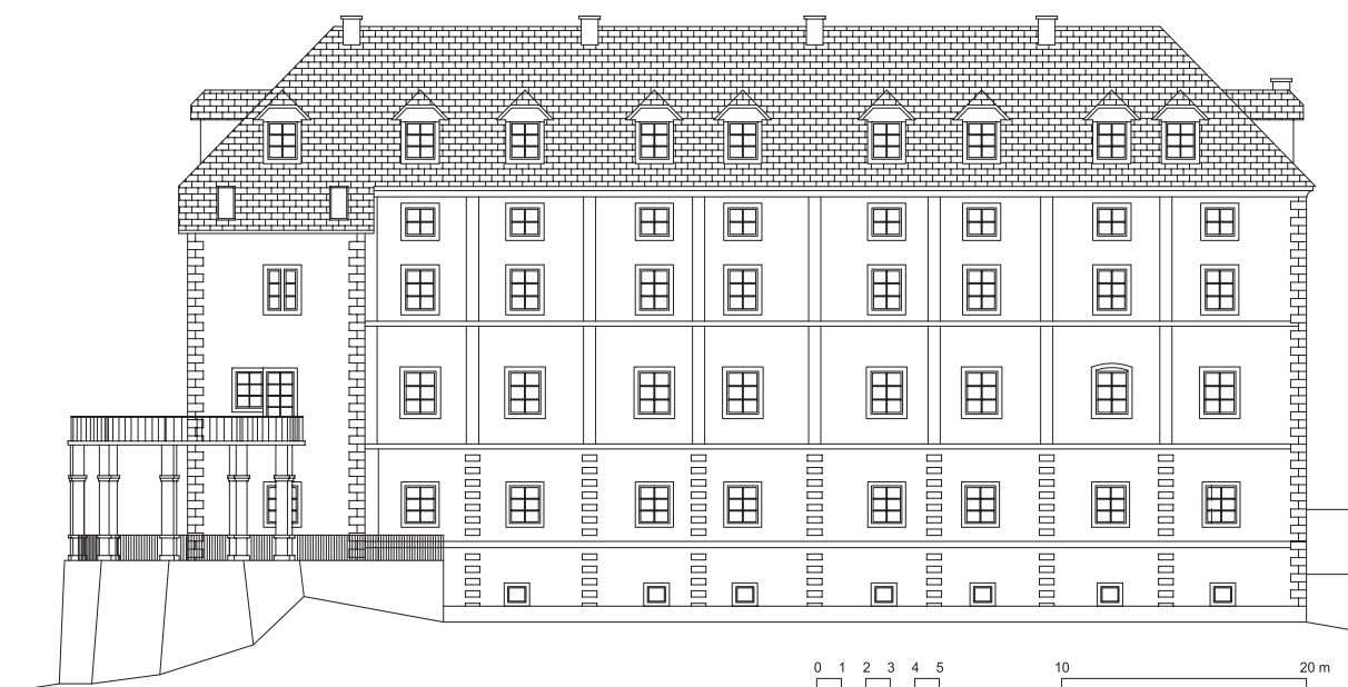
Izris proti dolini obrnjene severovzhodne fasade dvorca Turn v Šoštanju (risal: Igor Sapač, 2021).
