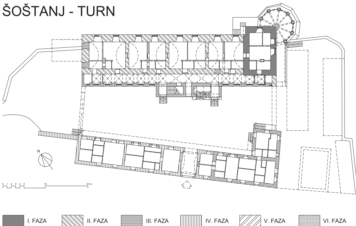
Tloris pritličja dvorca Turn v Šoštanju z vrisanimi fazami stavbnega razvoja ter črtkano označenimi porušenimi deli (risal: Igor Sapač, 2021).
