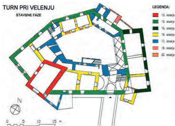
Tloris pritličja Turna pri Velenju z vrisanimi fazami stavbnega razvoja in z rdeče označenim zidovjem prvotnega stolpastega dvora iz 13. stoletja (risal: Igor Sapač, 2007, na podlagi starejšega posnetka).
