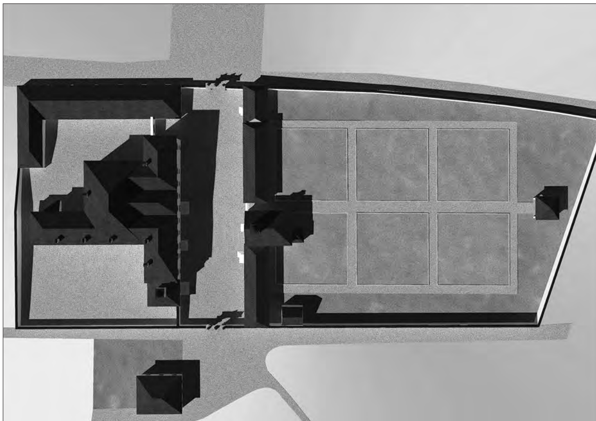
Kompleks dvorca Šoštanj po prenovi in razširitvi med letoma 1658 in 1681. Navpični pogled iz zraka. Računalniška studija. Poskus rekonstrukcije (izdelale Nastja Gorišek, Karin Pristovnik in Patricija Korez na podlagi risb Igorja Sapača, 2021).
