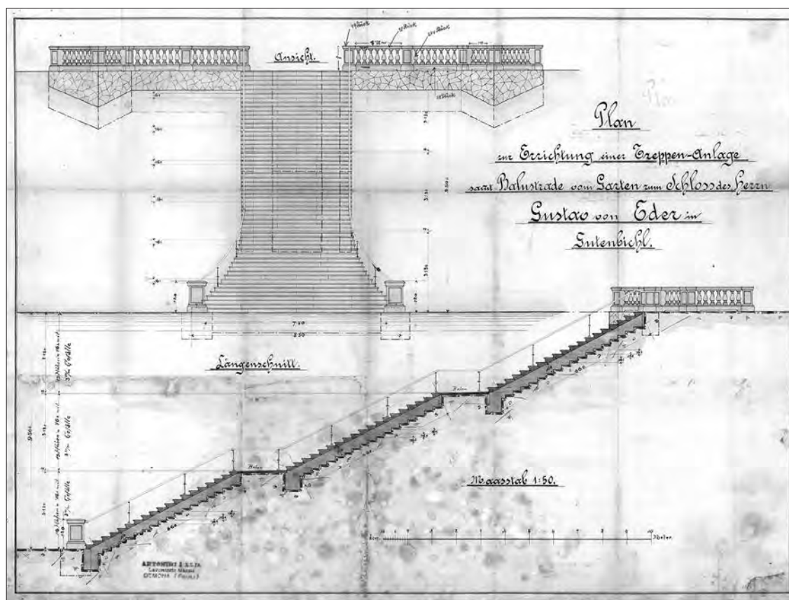
Načrt dvorca Gutenbüchel arhitekta Alfreda Kellerja iz leta 1926.
