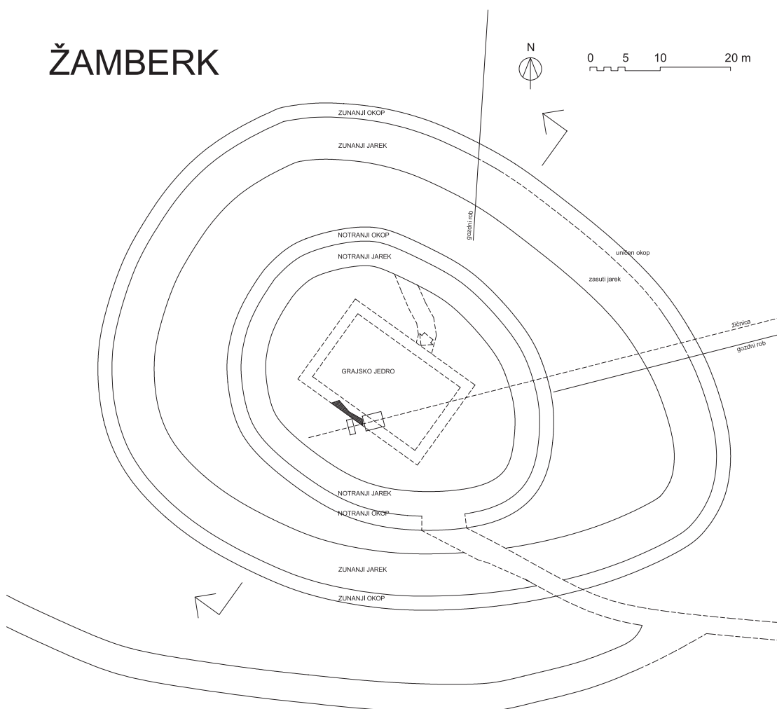
Tloris kompleksa nekdanjega gradu Žamberk s poskusom rekonstrukcije osnovne pravokotne tlorisne zasnove grajskega jedra (risal: Igor Sapač, 2021).
