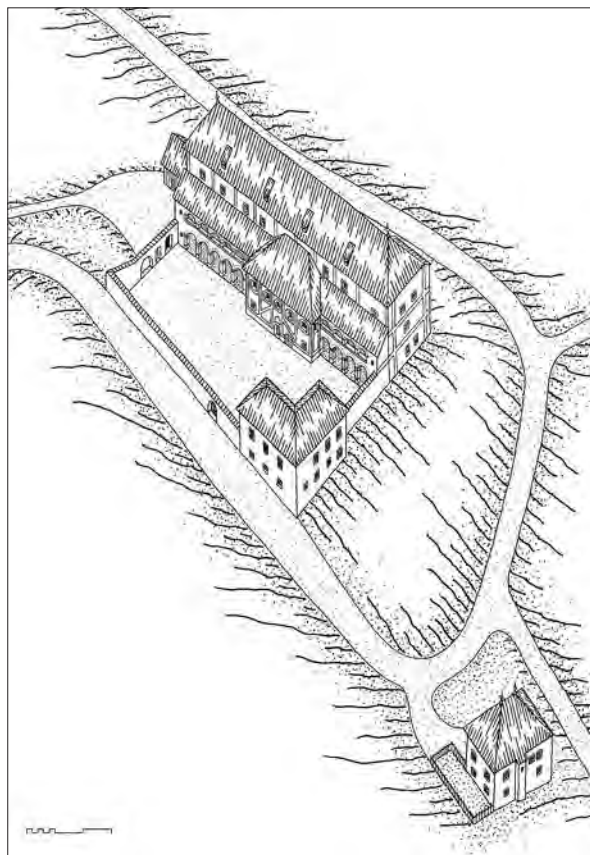
Dvorec Turn okoli leta 1790 (levo) in okoli leta 1880 (desno). Poskus rekonstrukcije. Aksonometrični študiji (risal: Igor Sapač, 2021).
