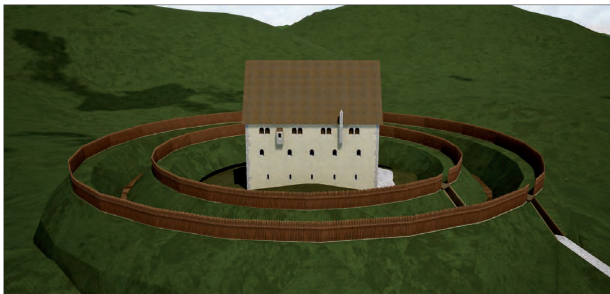
Variantna poskusa hipotetične rekonstrukcije nekdanje podobe gradu Žamberk. Pogled iz zraka z jugozahodne strani. Računalniška študija (izdelali Maja Žunkovič in Kaja Maroh na podlagi risb Igorja Sapača, 2021).
