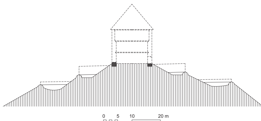
Prerez proti severozahodu lokacije gradu Žamberk s črtkano vrisanimi domnevnimi nekdanjimi višinami posameznih stavbnih delov (risal: Igor Sapač, 2016).
