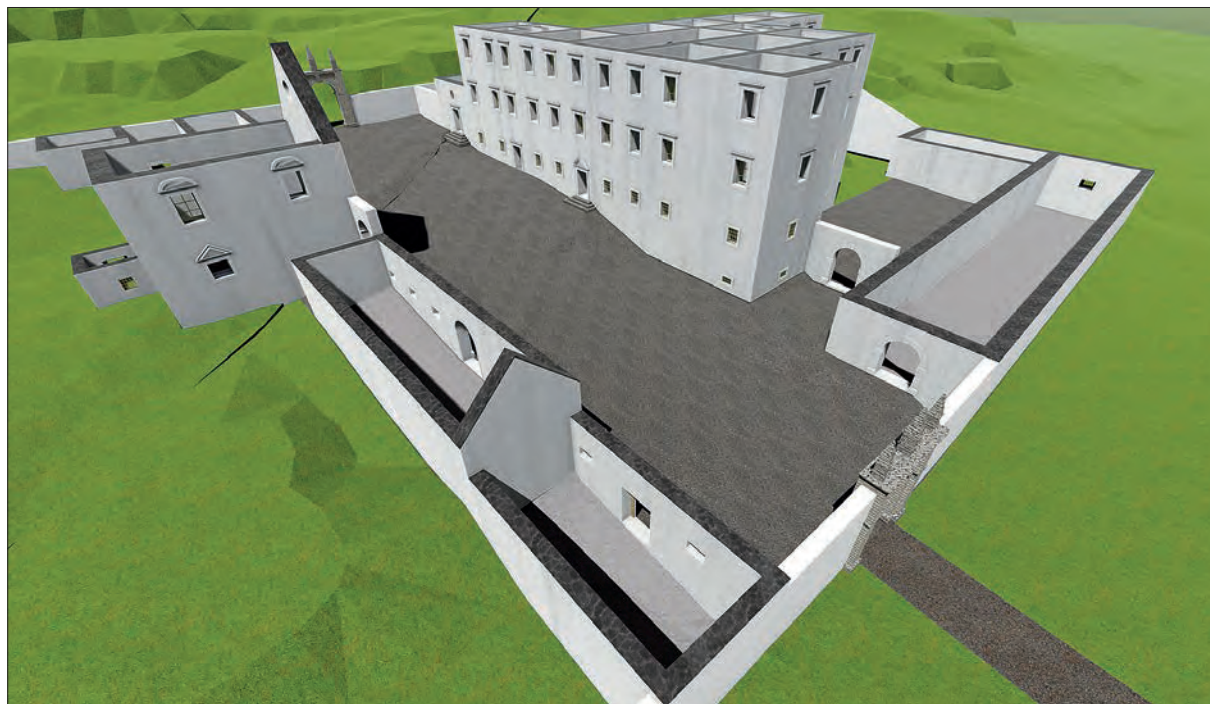
Pogled na kompleks dvorca Šoštanj iz zraka z vzhodne strani po požaru leta 1734. Računalniška študija. Poskus rekonstrukcije (izdelali Teodor Pagon, Jurij Petek in Uroš Polh na podlagi risb Igorja Sapača, 2021).
